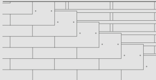
Recouvrement double
